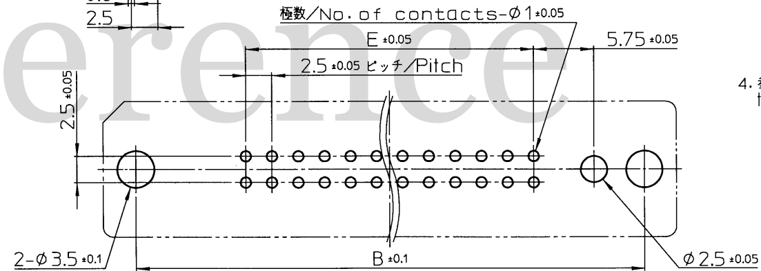
参考基板設計要領(コネクタ搭載面) A reference drawing of P.W.B.(connector mounting side)
