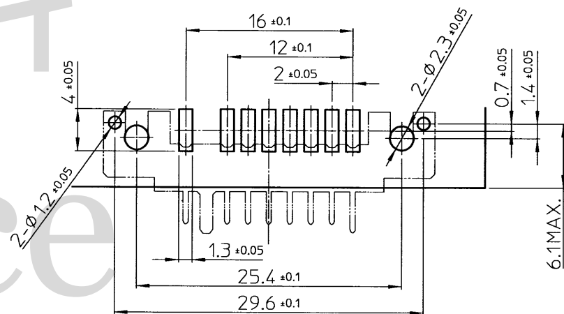
(コネクタ搭載面) 参考基板設計要領
