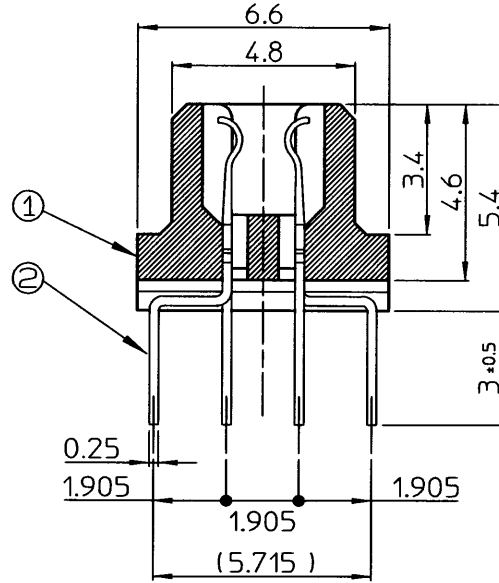
X-X'断面(5:1)
