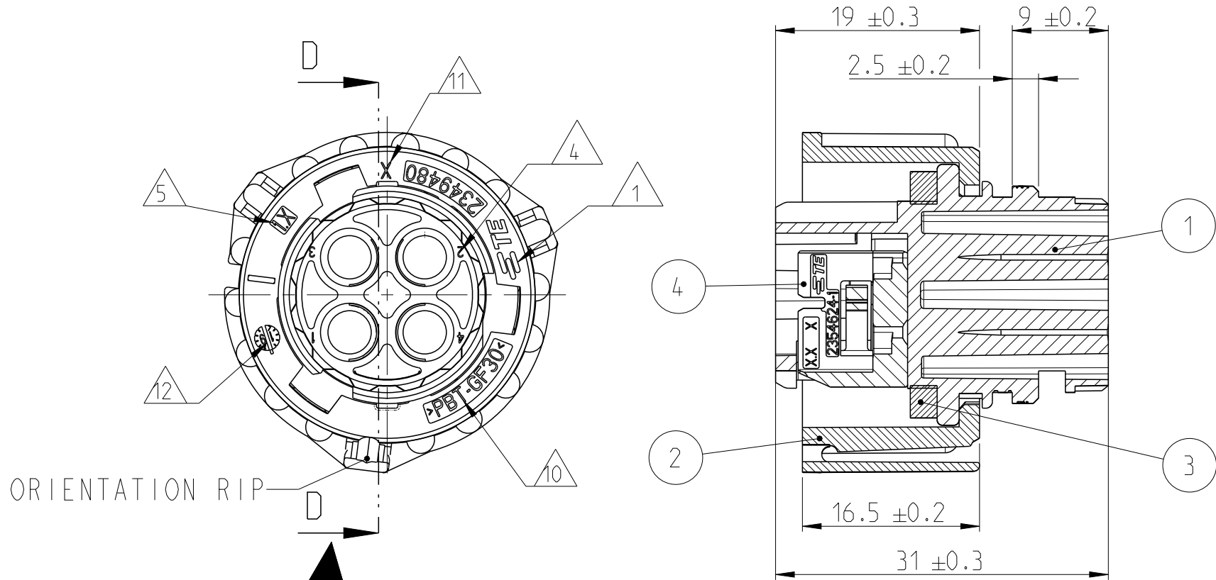
SECTION D-D
