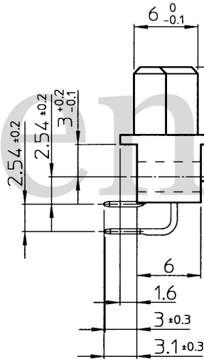
嵌合寸法関係図
