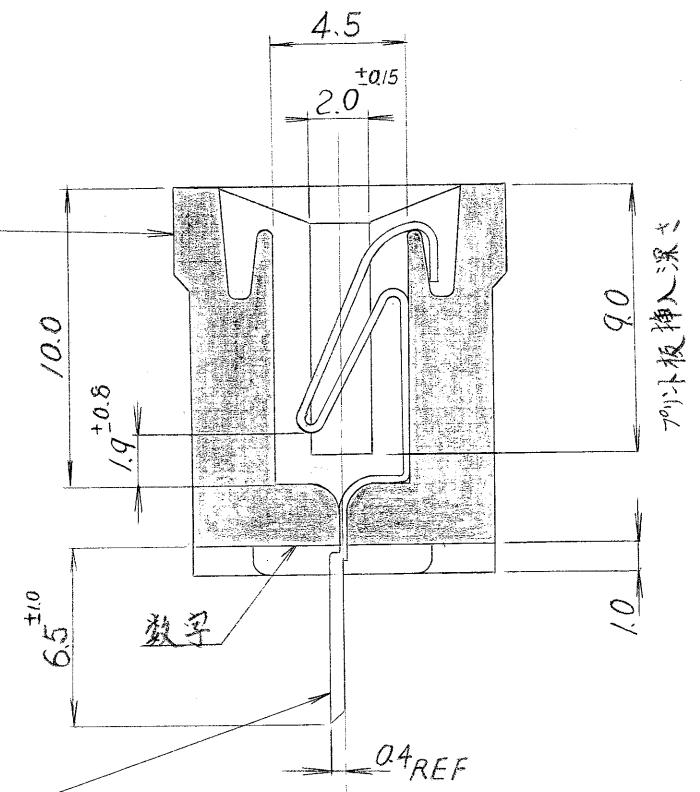
X-X 断面細詳図 尺度 4/1
