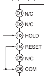
端子台型 〈1〉〈3〉
