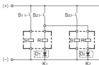
置位线圈、重置线圈的连接电路
