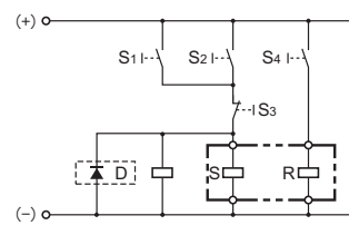
在置位线圈上并联其它的继电线圈的电路
