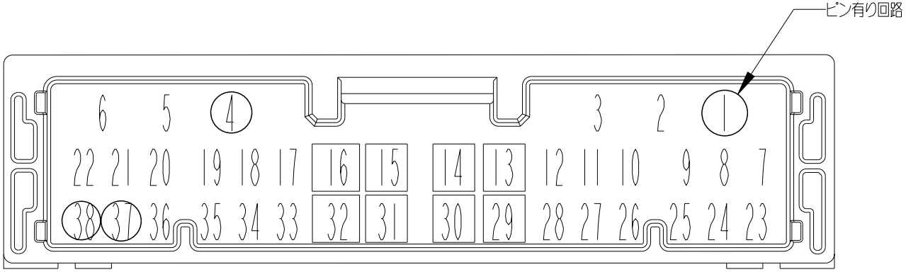
FIG. 1 CIRCUIT NUMBERS/回路番号
