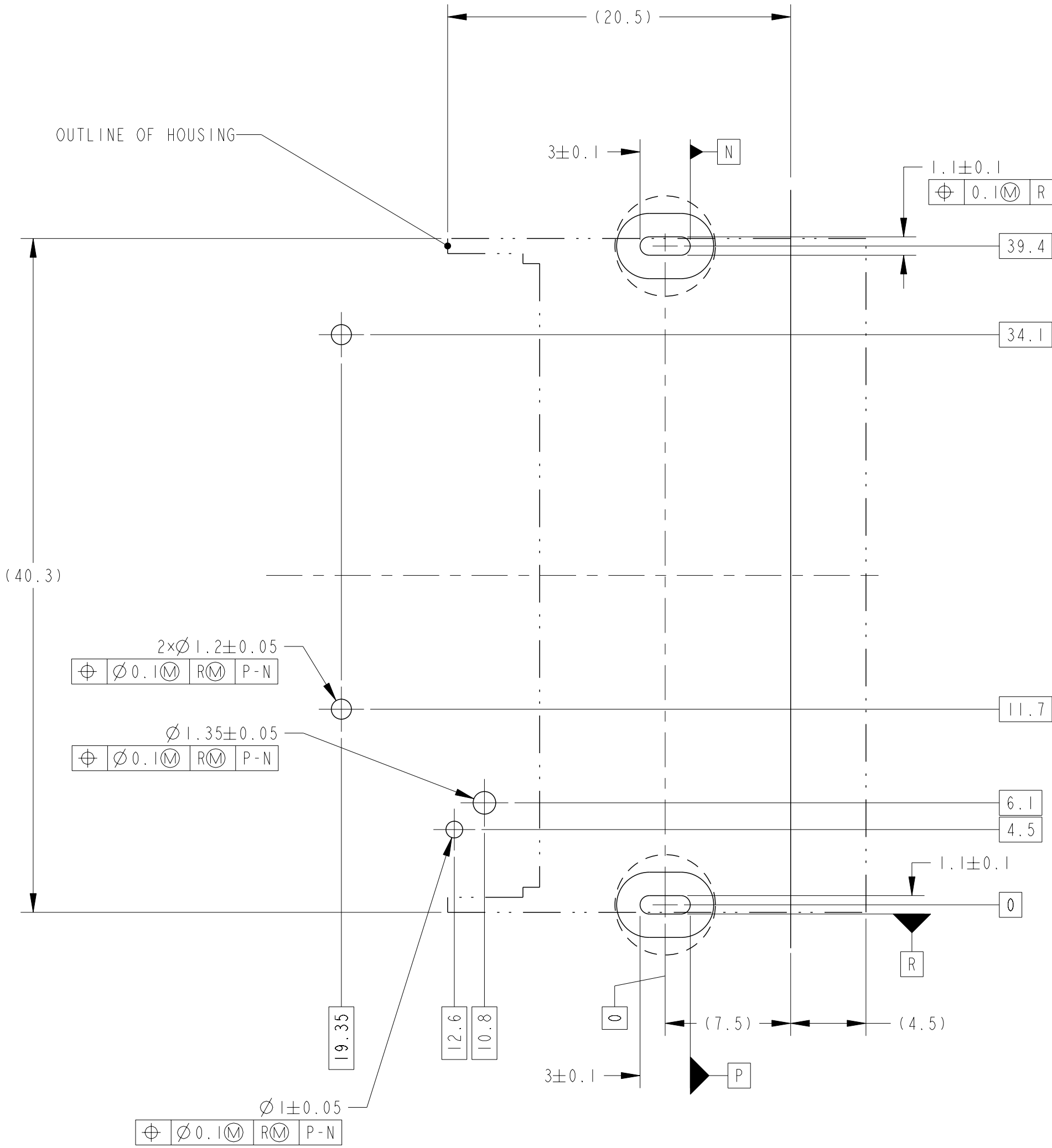
FIG. 3 推奨プリント基板取付寸法図 RECOMMEND DIMENSION FOR P.C.B.
