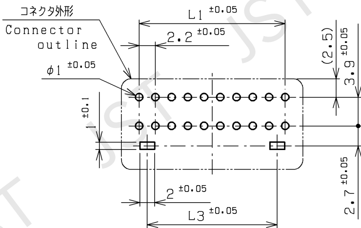
8P、12P、20P推奨基板穴寸法 (コネクタ装着側) 8P、12P、20P Recommendable P.C. Board hole layout (connector mounted side)
