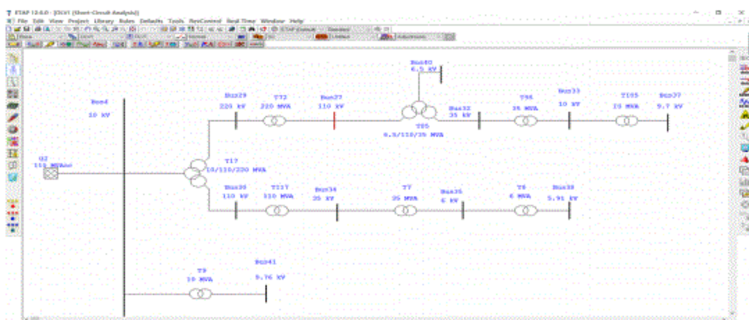
图 4.5 设置故障的单线图
