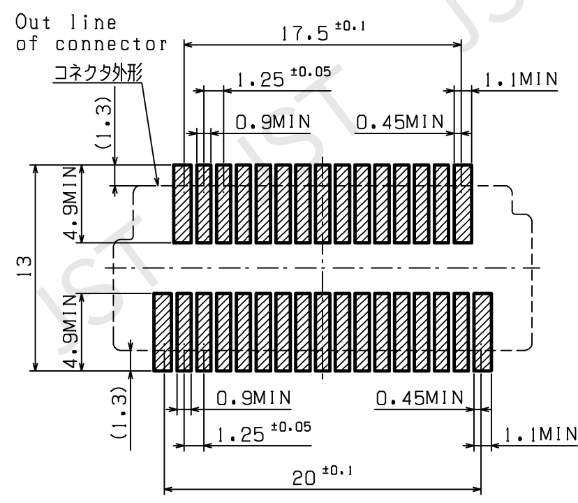
パターンレイアウト (推奨) Recommended pattern layout
