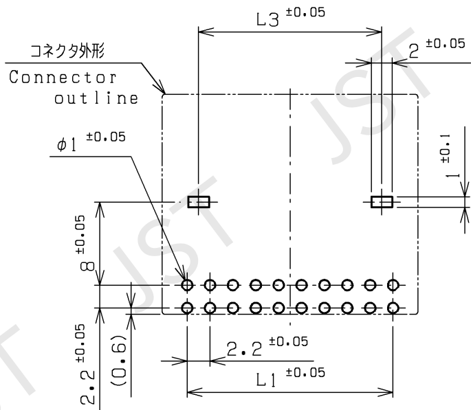
12P、20P推奨基板寸法 (コネクタ装着側) 12P、20P Recommendable P.C. Board hole layout (connector mounted side)
