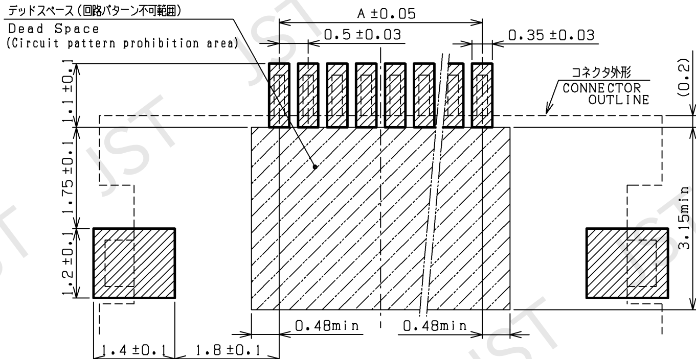
参考基板レイアウト (コネクタ搭載面) REFERENCE PC BOARD LAYOUT (FROM TOP VIEW)
