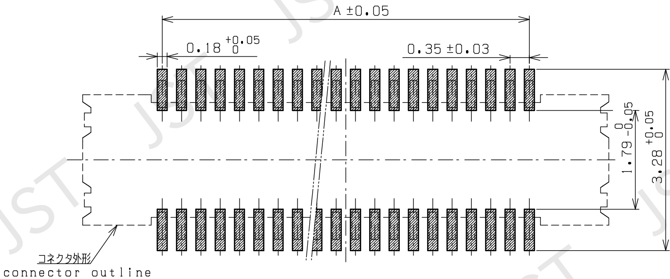
推奨基板レイアウト RECOMMENDABLE P.C.B LAYOUT
