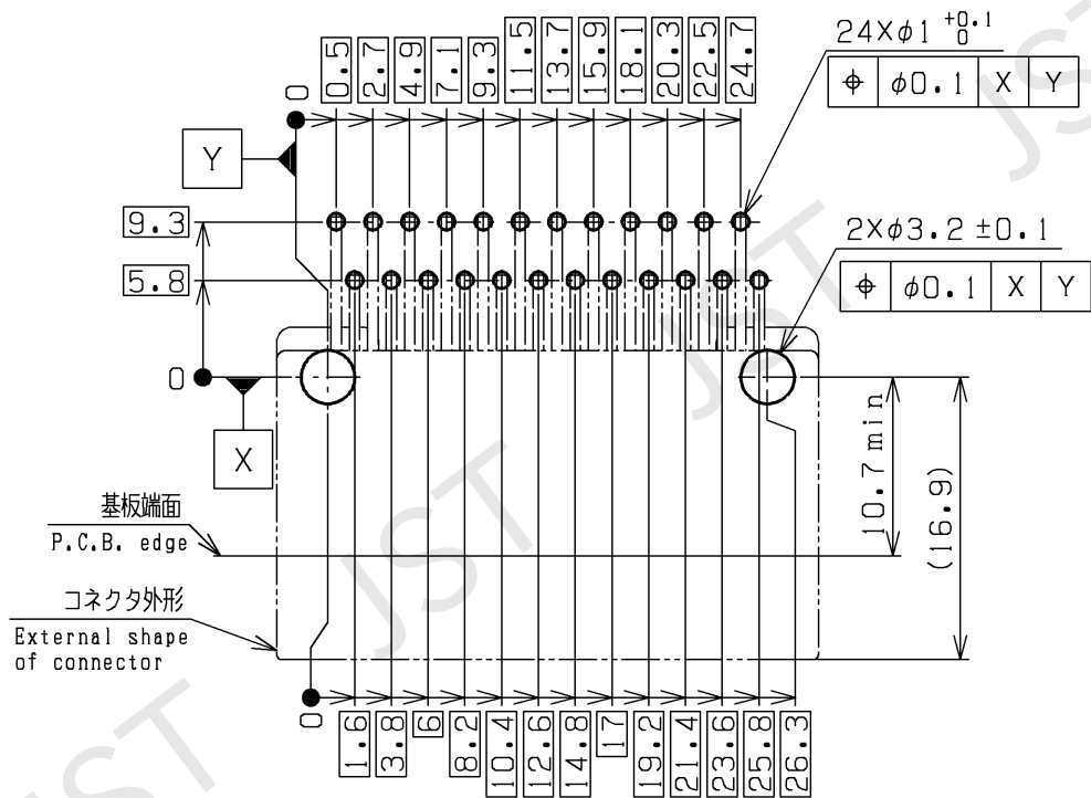
推奨パターンレイアウト/ P.C.B. layout ＜コネクタ装着側/ View from connector mounting side＞
