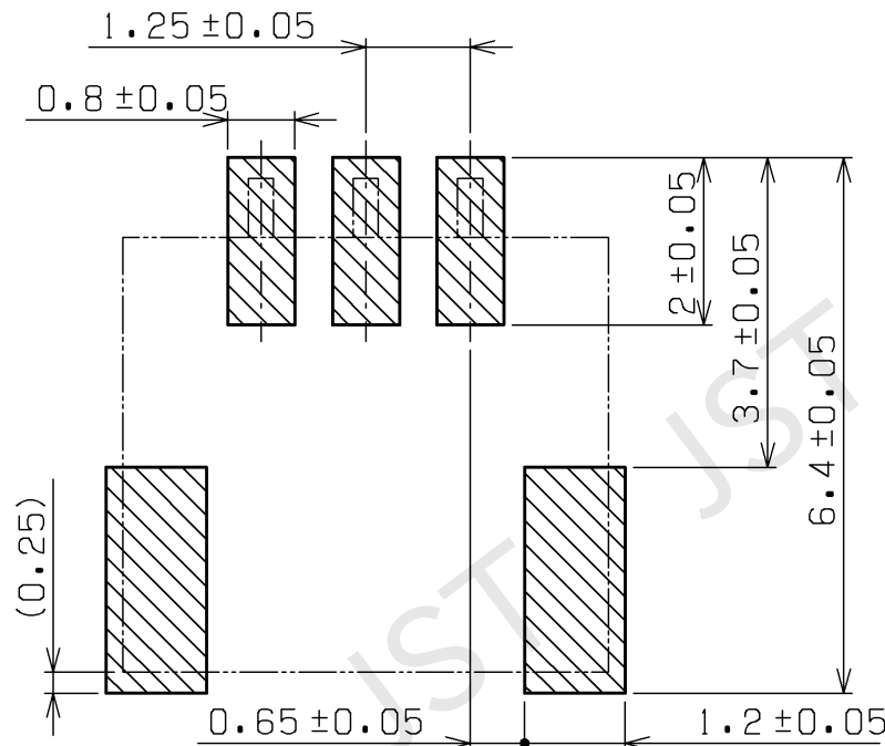
基板レイアウト参考寸法 P.C.Board Layout
