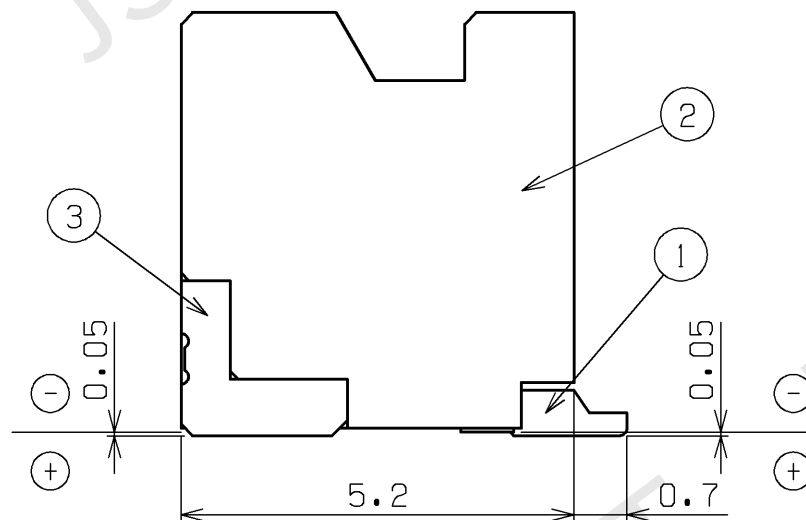
基板レイアウト参考寸法 P.C.Board Layout
