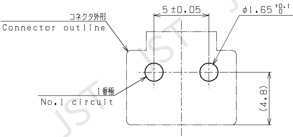
推奨基板穴レイアウト (コネクタ装着側) Recommendable P.C. Board layout (Connector mounted side)
